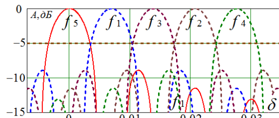
Рис. 7. АЧХ вхідного/вихідного перетворювача з псевдоортогональним частотним кодуванням
