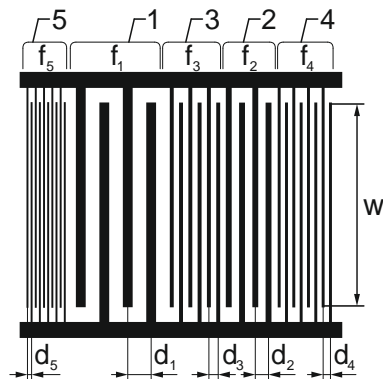
Рис. 1. ПАХ-перетворювач з 5-ма частотами кодування
