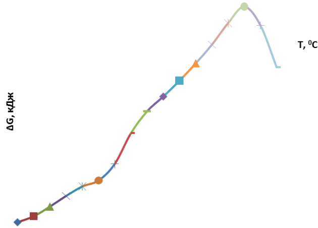
Рисунок 2. Зависимость \Delta G системы Fe_2P + Al = AlP + 2Fe от температуры
