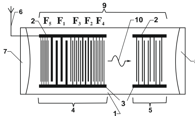
Рис.3. Конструкція радіомітки на ПАХ
