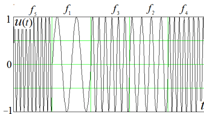
Рис. 2. Сигнал радіозапиту, узгоджений до вхідного перетворювача
