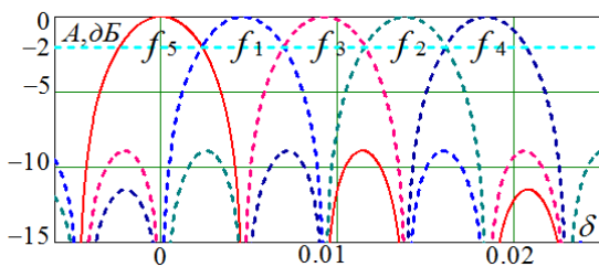
Рис. 6. АЧХ вхідного/вихідного перетворювача з ортогональним частотним кодуванням
