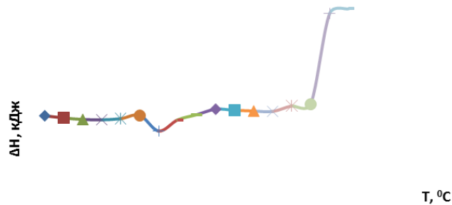
Рисунок 3. Зависимость \Delta H системы Fe_3P + Al = AlP + 3Fe от температуры
