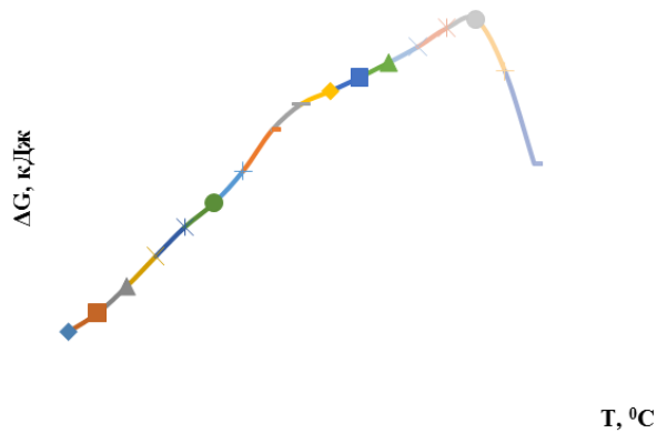
Рисунок 4. Зависимость \Delta G системы Fe_3P + Al = AlP + 3Fe от температуры
