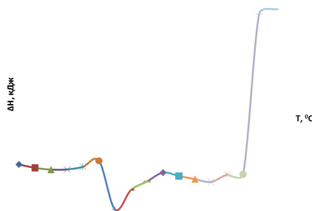
Рисунок 1. Зависимость \Delta H системы Fe_2P + Al = AlP + 2 Fe от температуры
