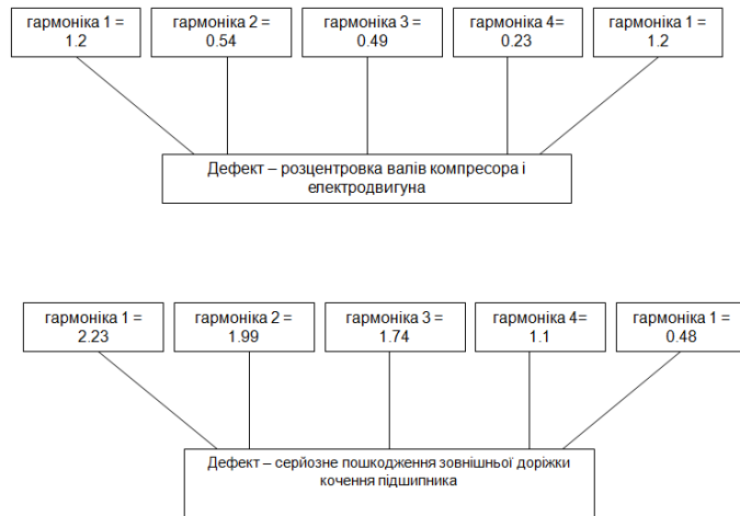
Рисунок 6 - Схема побудови внутрішніх правил
