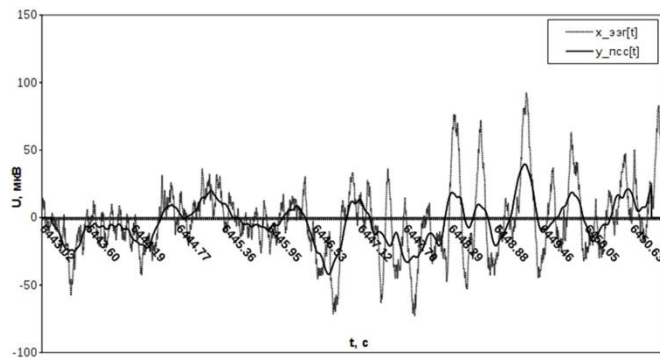
Рисунок 5 – Результат низькочастотної фільтрації ЕКГ при m=38
