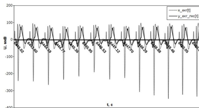
Рисунок 4 – Результат низькочастотної фільтрації ЕЕГ при m=60
