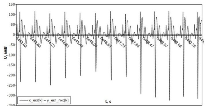
Рисунок 7 – Високочастотна складова сигналу ЕКГ
