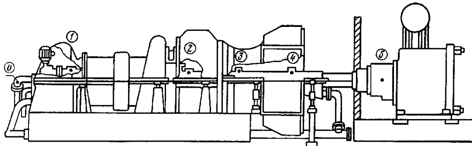
Рисунок 4 - Схема компресора з контрольними точками вимірювання
