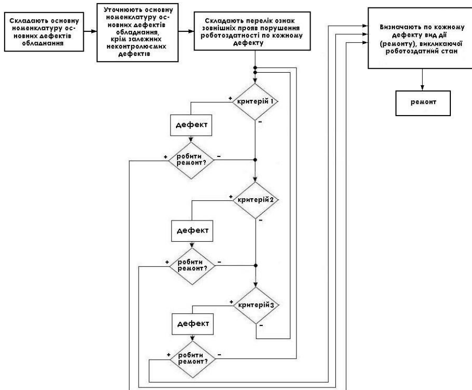
Рисунок 7 - Блок схема діагностування ГПА
