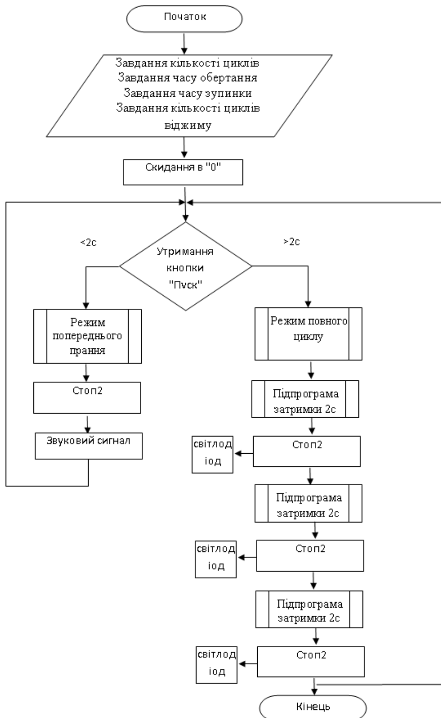
Рисунок 1 - Блок-схема алгоритму програми роботи контролера
