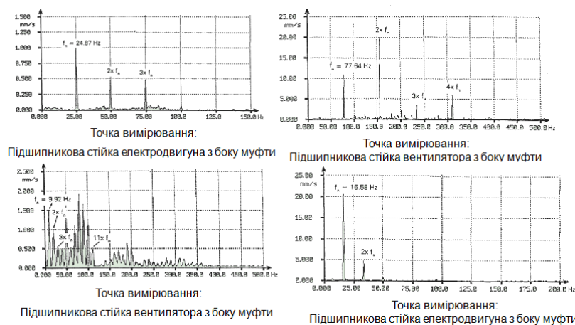
Рисунок 5 - Спектри віброшвидкості
