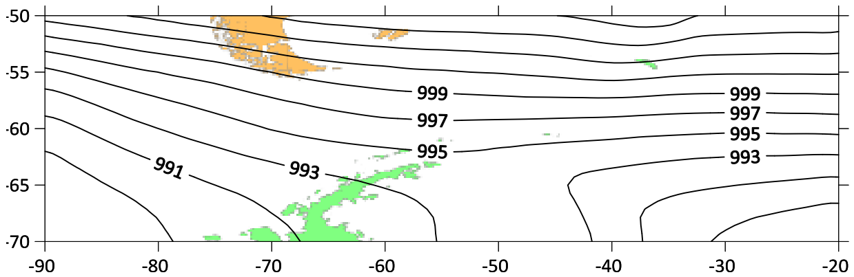
Рис. 2 Поле середніх значень приземного атмосферного тиску (липень)
