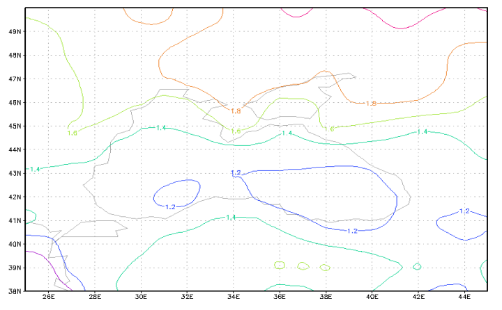
Рис. 4 Поле середніх квадратичних відхилів приземної температури повітря (липень)
