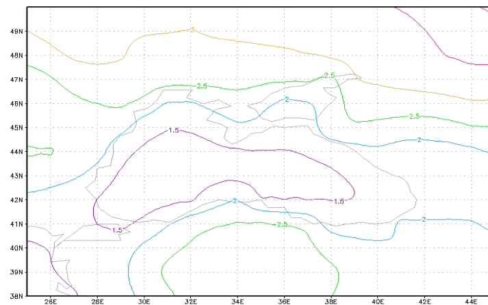
Рис. 3 Поле середніх квадратичних відхилів приземної температури повітря (січень)
