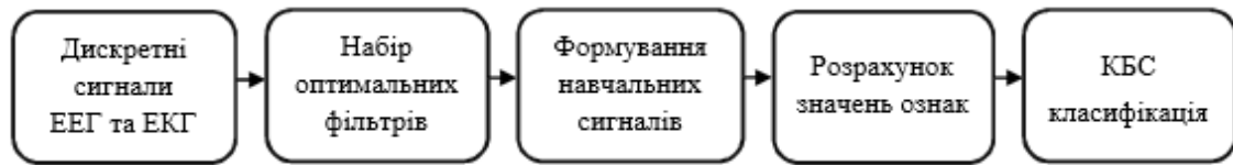
Рисунок 4.1 – Структура алгоритму
