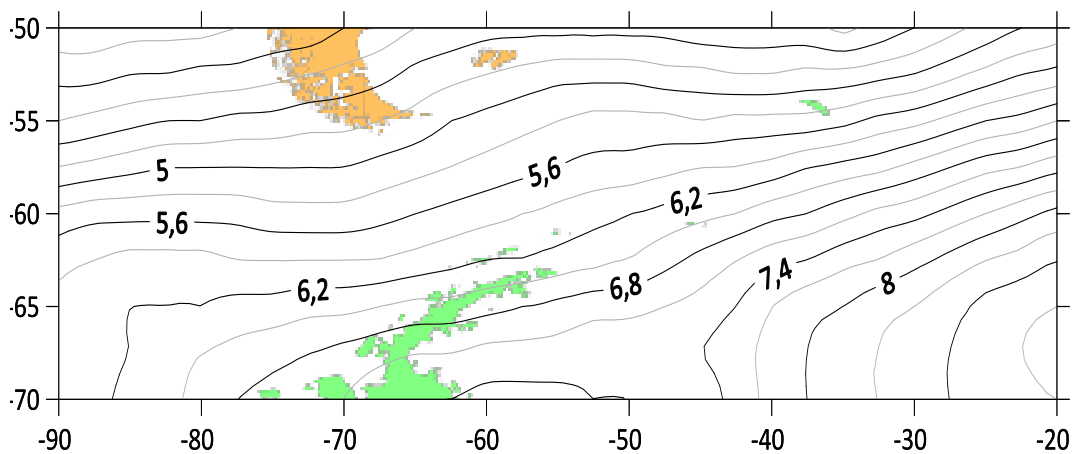
Рис. 4 Поле середніх квадратичних відхилів приземного атмосферного тиску (липень)
