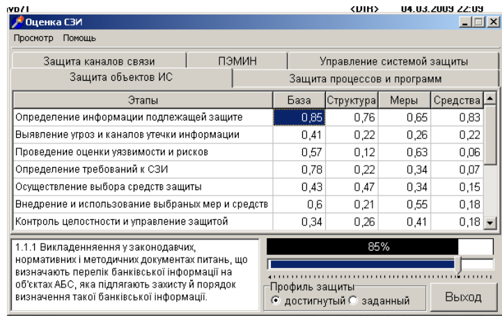
Рис. 1.2. Програмный продукт «Модель системной интеграции модулей защиты информации в АБС банку»
