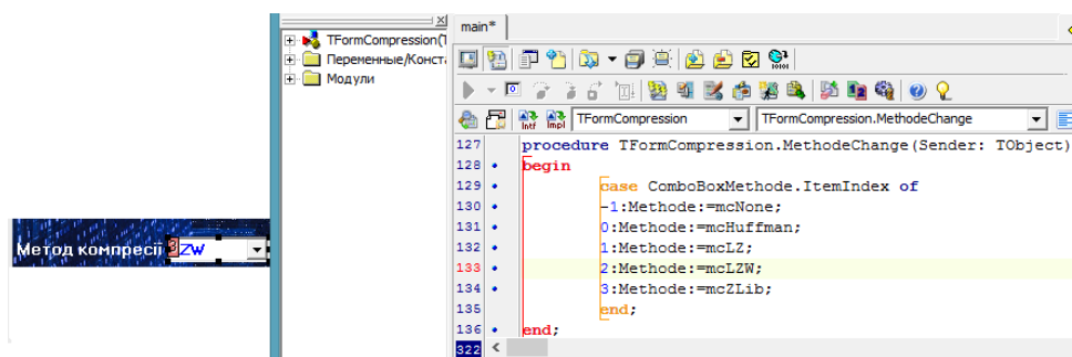
Рисунок 7 – Програмний код роботи компонента ComboBox
