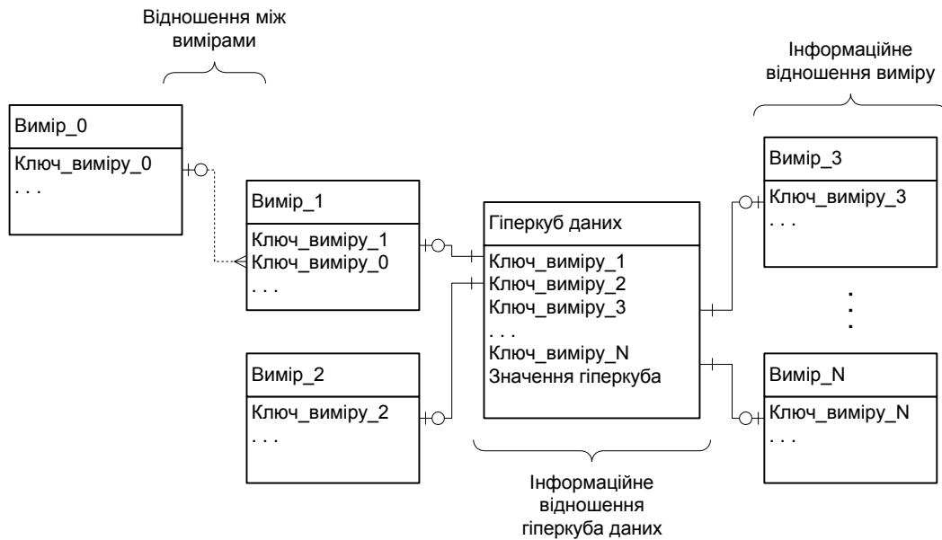
Рис.1. Схема гіперкуба даних
