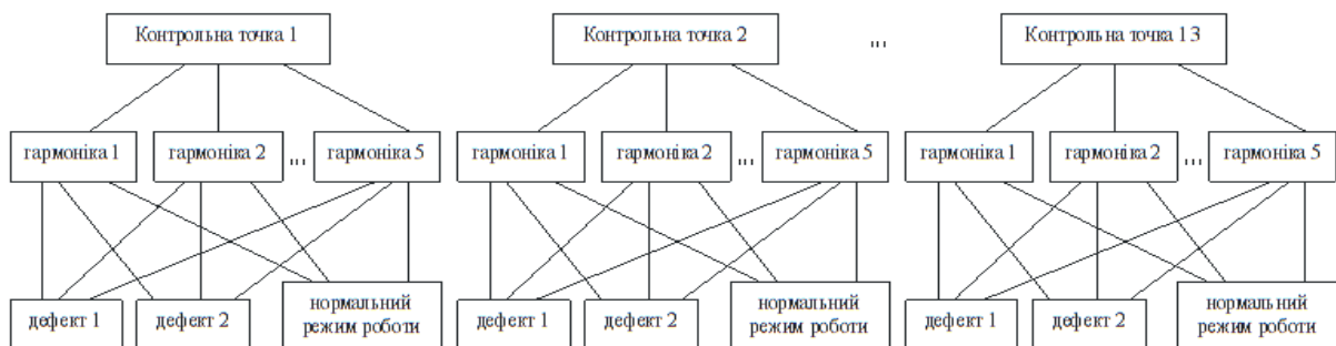
Рисунок 8 - Схема загальної структури експертної системи
