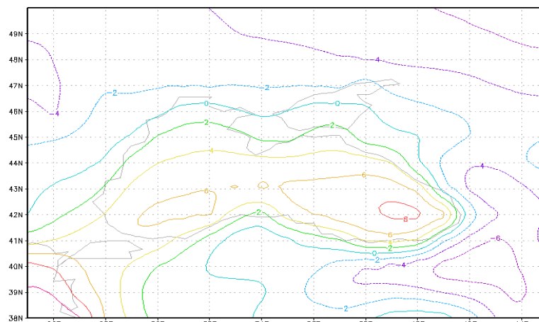
Рис. 2 Поле середніх значень приземної температури повітря (січень)
