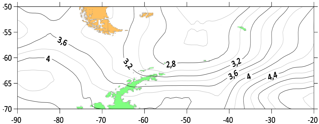
Рис. 3 Поле середніх квадратичних відхилів приземного атмосферного тиску (січень)
