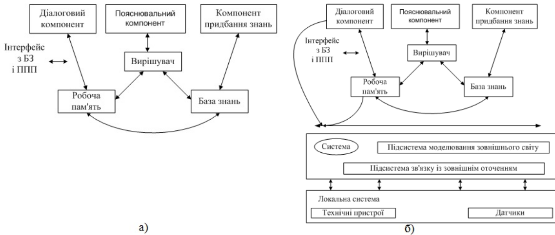
Рисунок 1 - Архітектура експертних систем а) статична, б) динамічна
