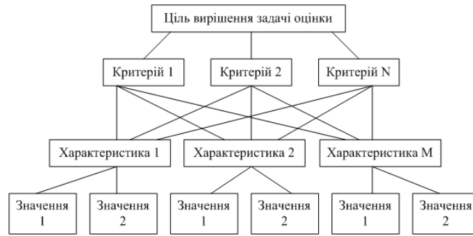
Рисунок 3 - Ієрархія бази знань в "ExPro"
